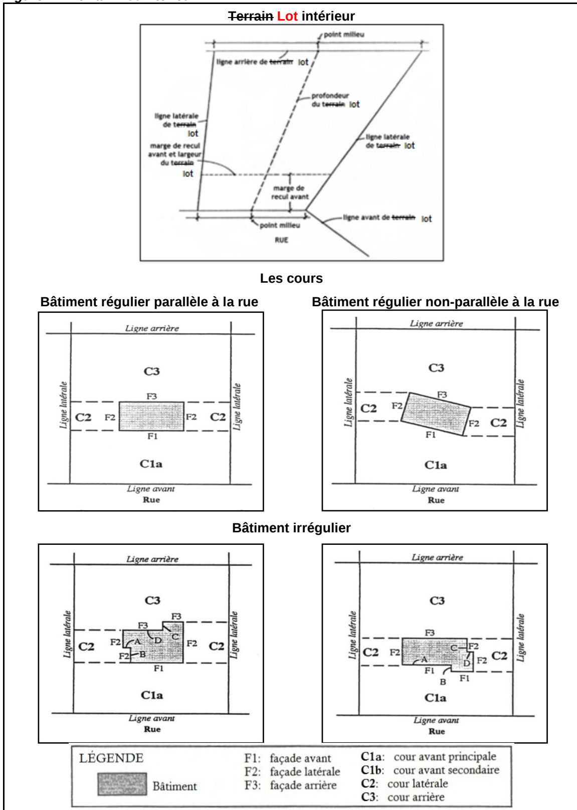
Figure 12 Terrain Lot intérieur
