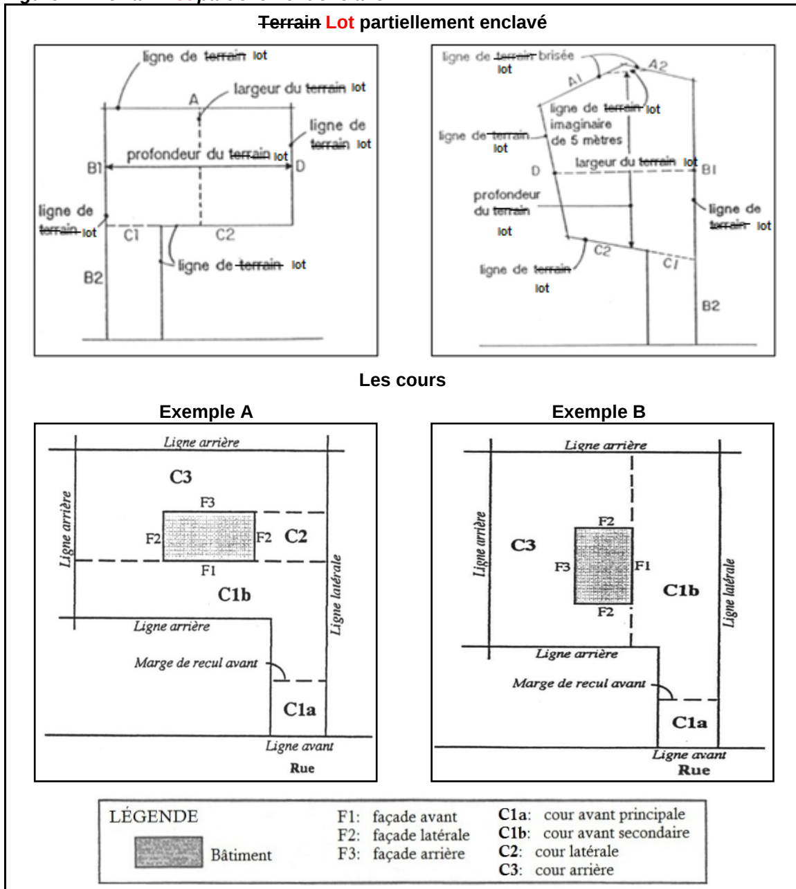
Figure 14 Terrain Lot partiellement enclavé
