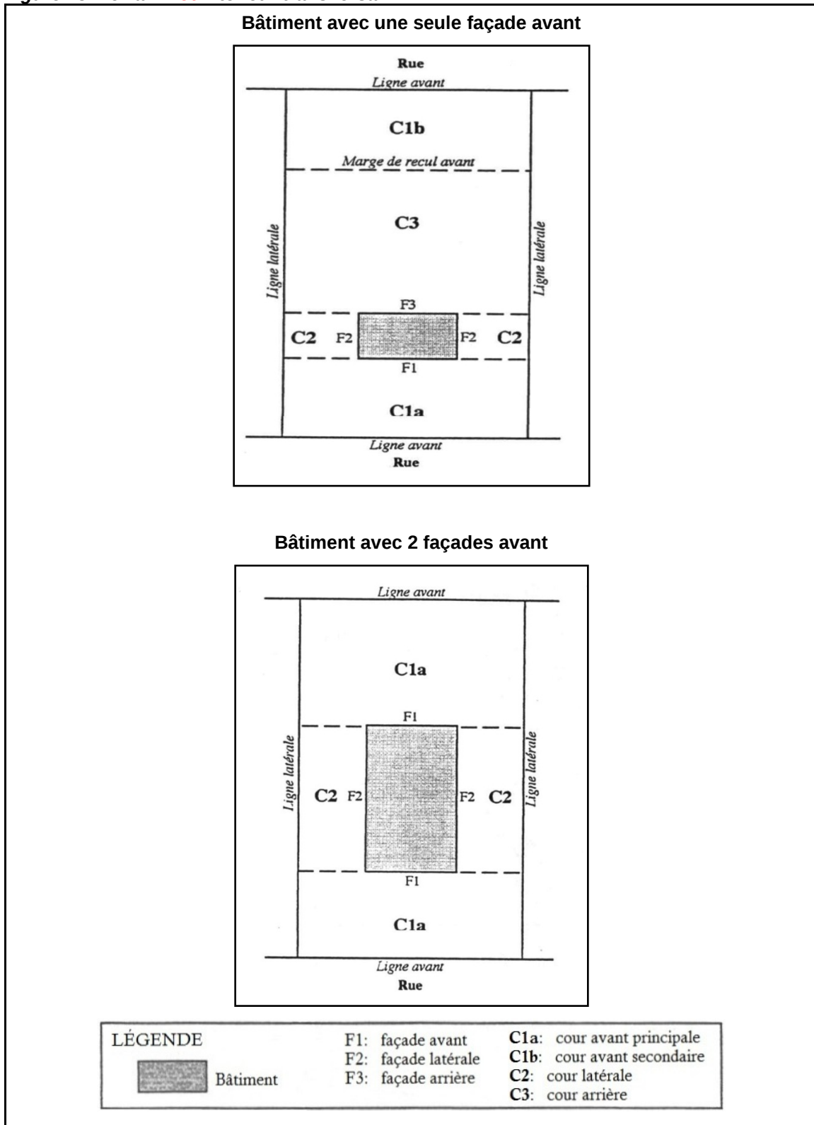
Figure 13 Terrain Lot intérieur transversal
