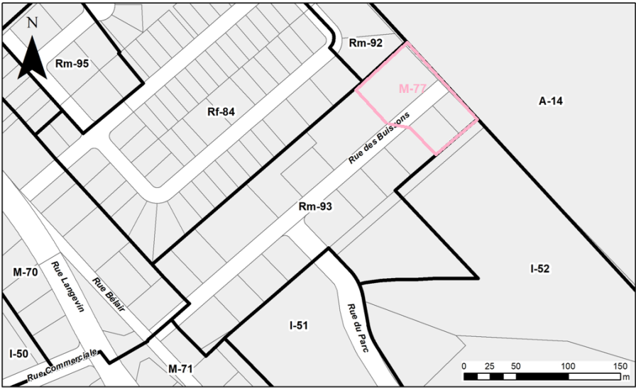
Après modification
